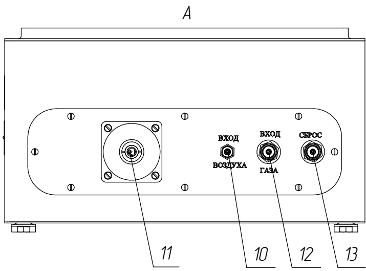
Рисунок 14 – Блок отбора пробы. Внешний вид
