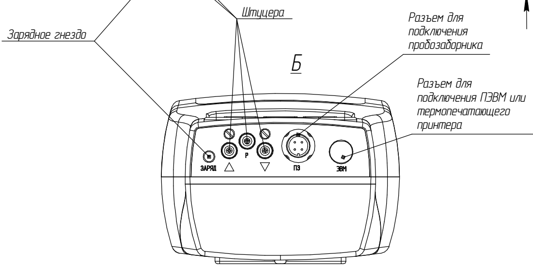
Рисунок 1.1 – Газоанализаторы АНКAT-310. Внешний вид
