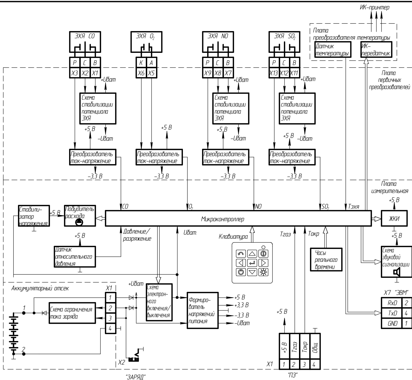
Рисунок 1.2 – Газоанализаторы АНКАТ-310. Функциональная схема
