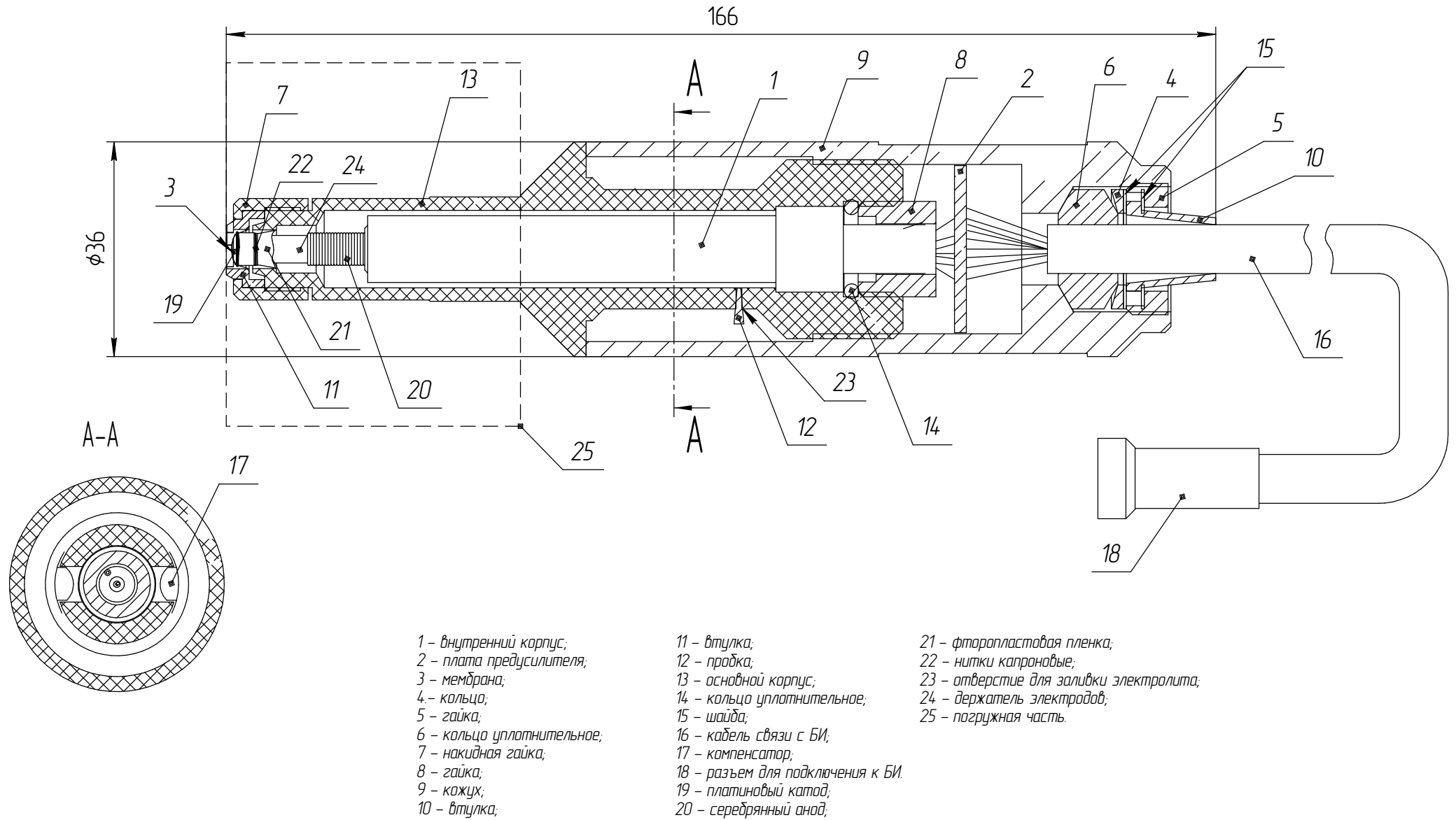
Рисунок 1.3 - Внешний вид и конструкция датчика
