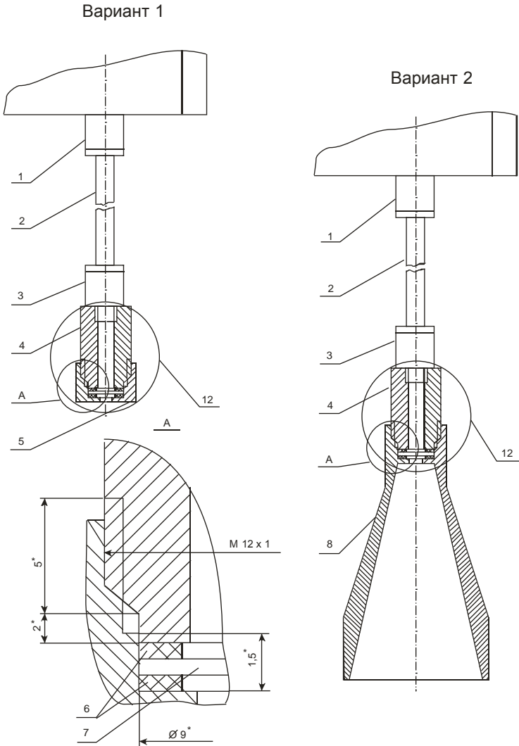
Рис. 7а. Проботборное устройство (вариант 1 и 2)
