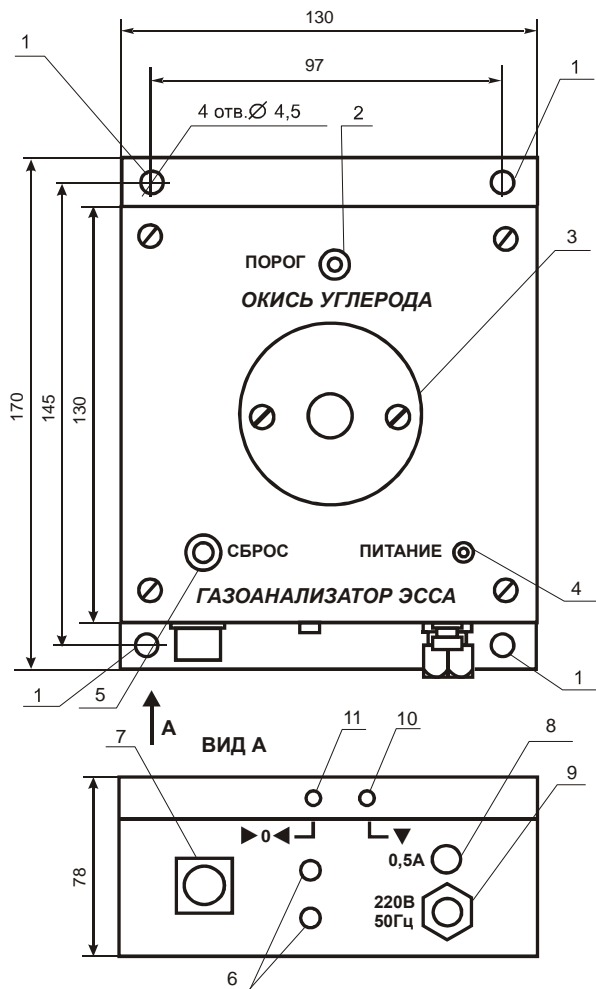
РИС. 1. БИС газоанализатора ЭССА - CO, габаритные и установочные размеры.
