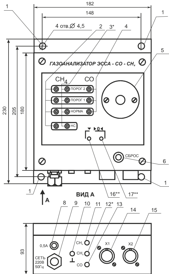
РИС. 2. БИС газоанализаторов ЭССА - СО - СН 4 (/2) габаритные и установочные размеры.
